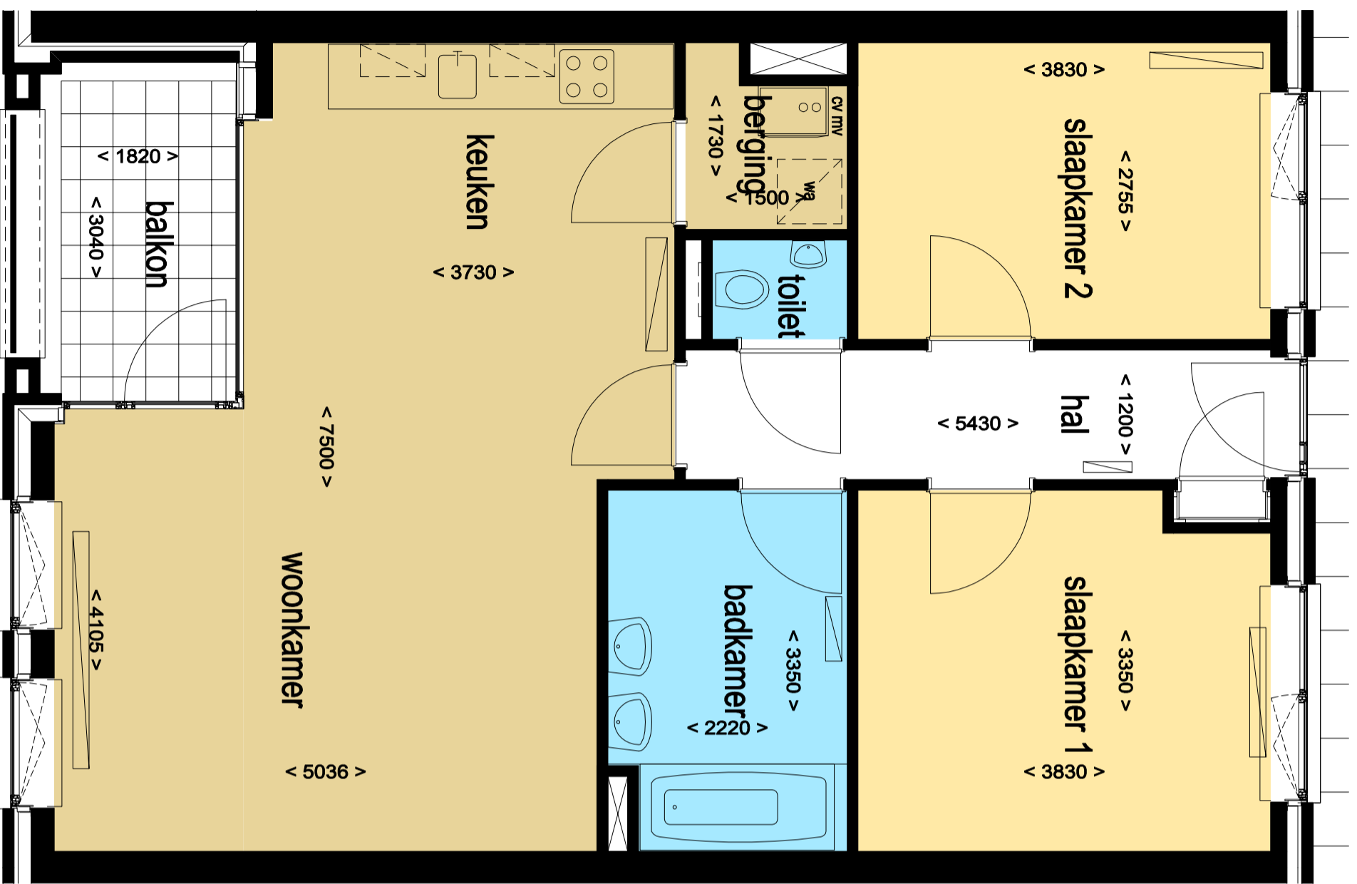
APPARTEMENT 1.2 - Type A(s)
