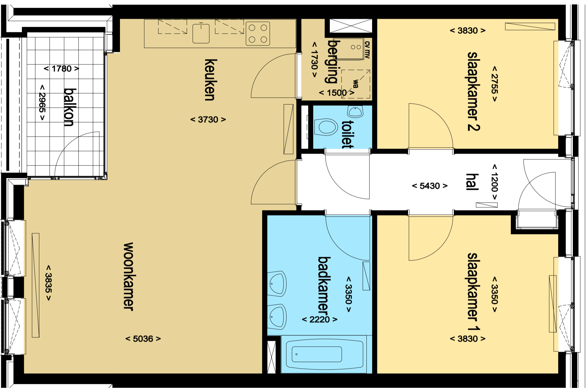
APPARTEMENT 2.3 - Type A(s)
