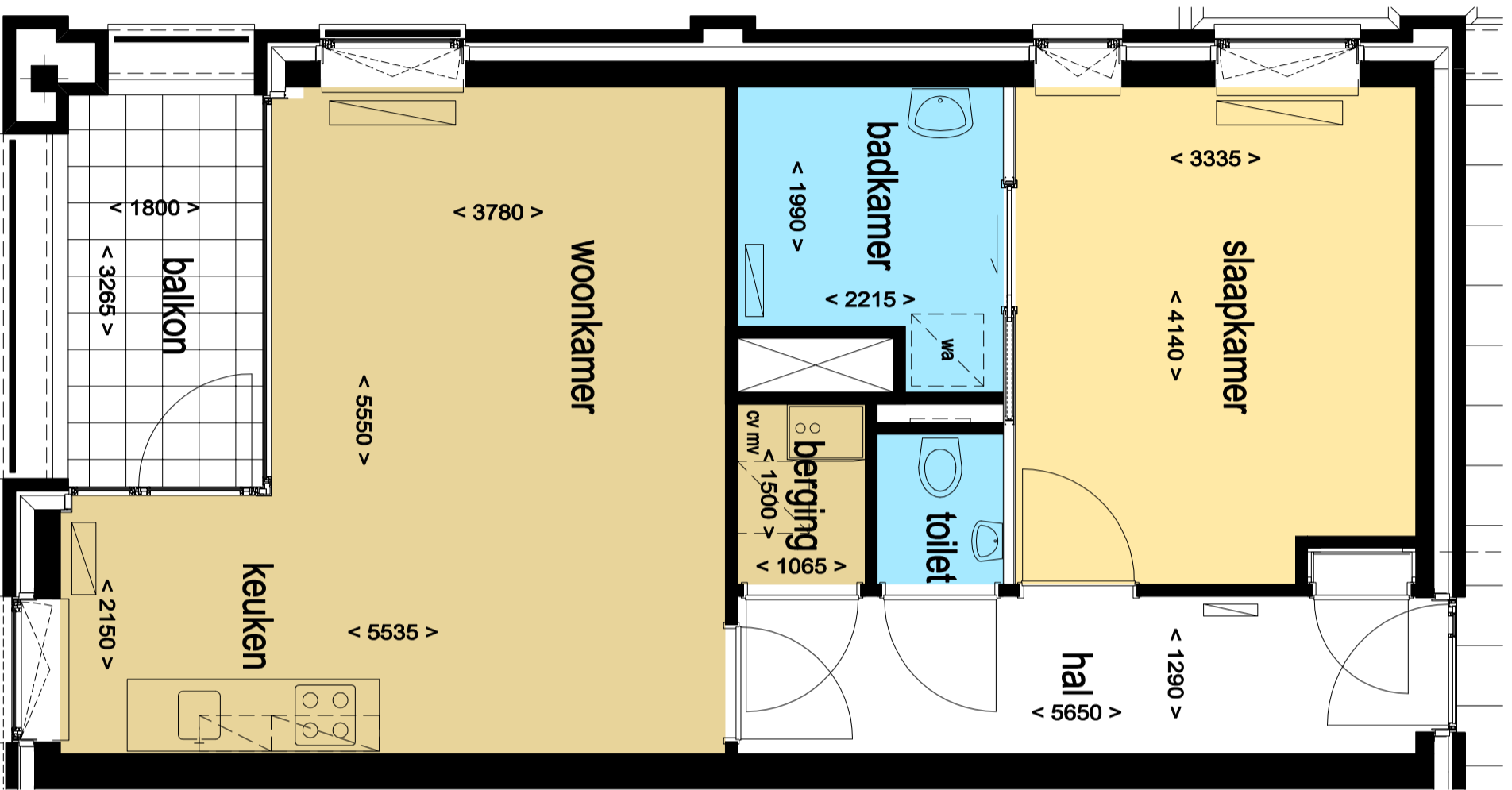
APPARTEMENT 1.7 - Type E(s)
