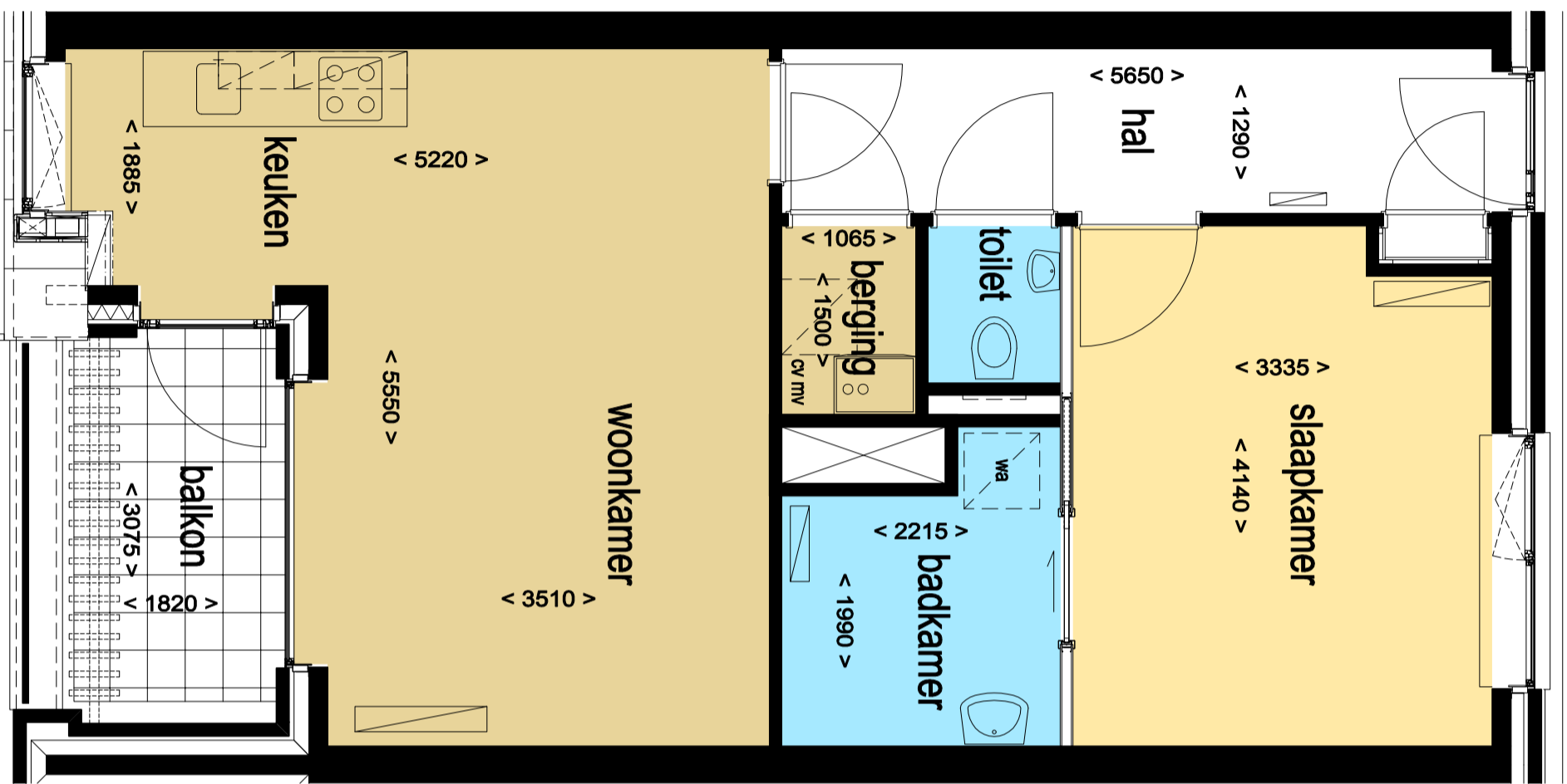
APPARTEMENT 2.4 - Type E1
