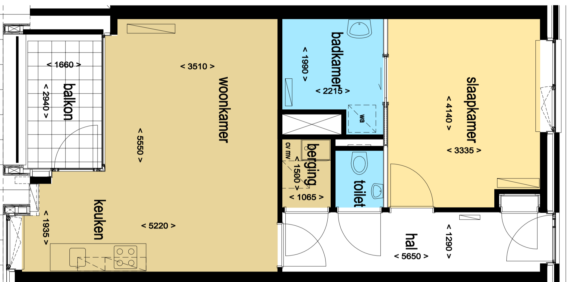
APPARTEMENT 2.5 - Type E(s)
